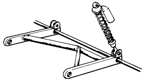
Fig. 5. Exempel på en hjulupphängning bak (länkarm med stag, fjäder och stötdämpare).
